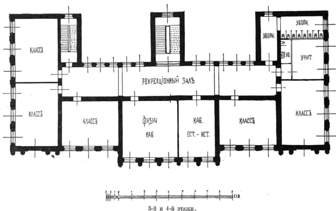
Рисунок 4. Исторический план 3-4 этажей.
